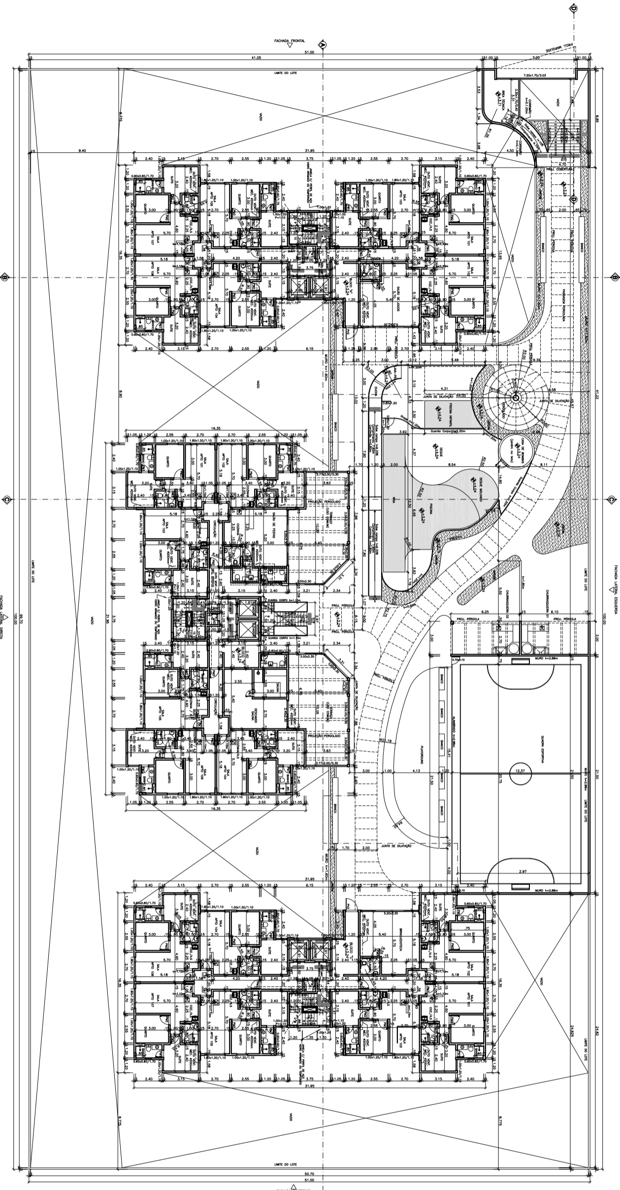
PLANTA BAIVA - 1º PAVIMENTO (LAZER)
